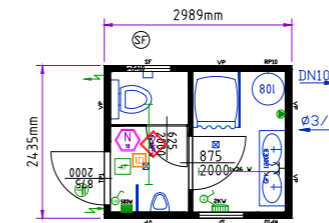
Sanitärcontainer 10'
