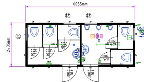
WC-Container Damen/Herren 20'
