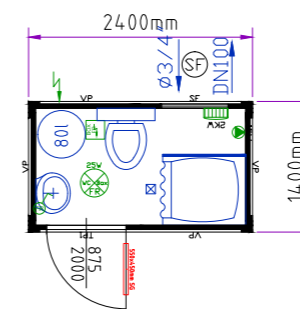
WC-Dusch-Container 8'
