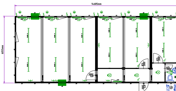
Büro- und Sanitärcontainer 6er-Anlage
