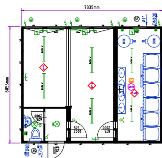
Büro- und Sanitärcontainer 3er-Anlage
