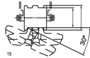
19 OPTIMALE KETTENFÜHRUNG
